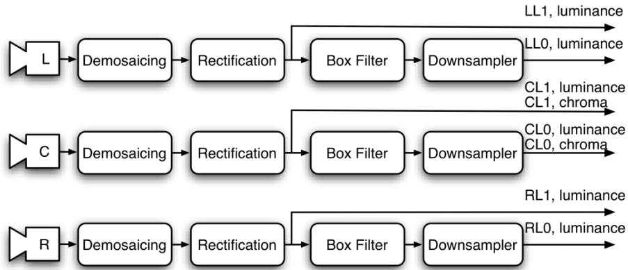
Fig. 10. Pre-processing module
