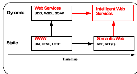
Fig. 1. Semantic Web enabled Web Services
