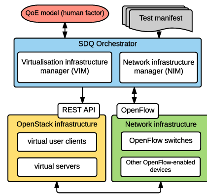
Fig. 1. SDQ framework
