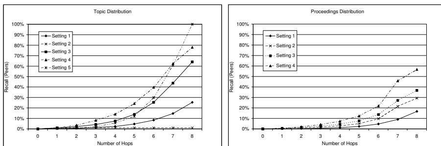
Fig. 3. Recall_{Peers}
