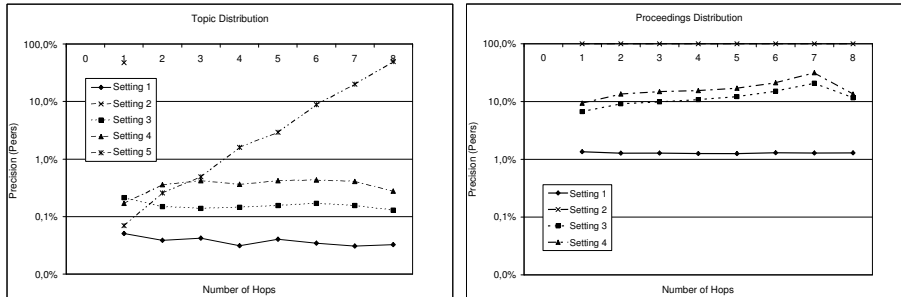
Fig. 2. Precision_{Peers}
