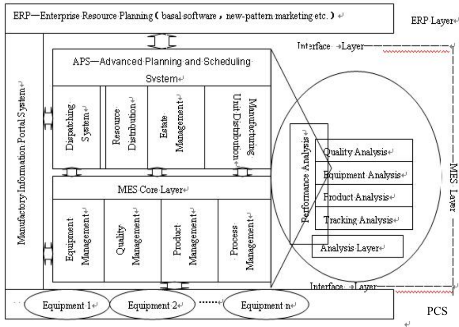
Figure. 5 MES Function Structure
