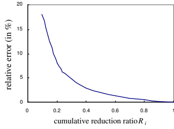
Fig. 2. Error Function g(R_i)
