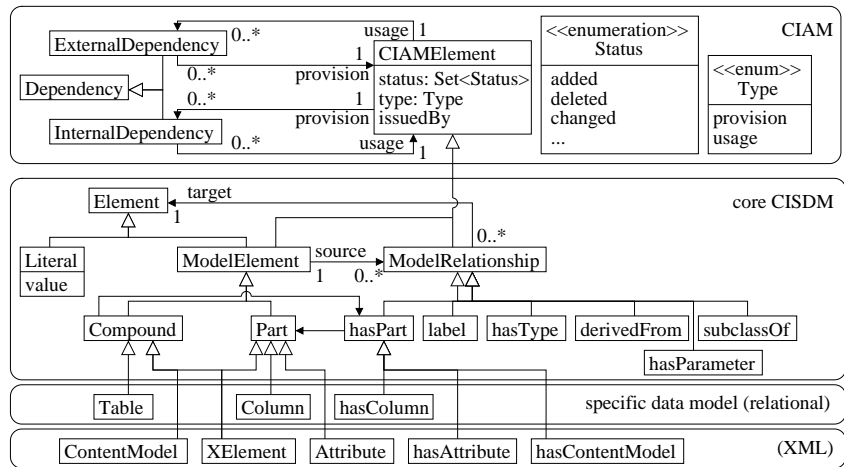
Fig. 4. Caro meta-models
